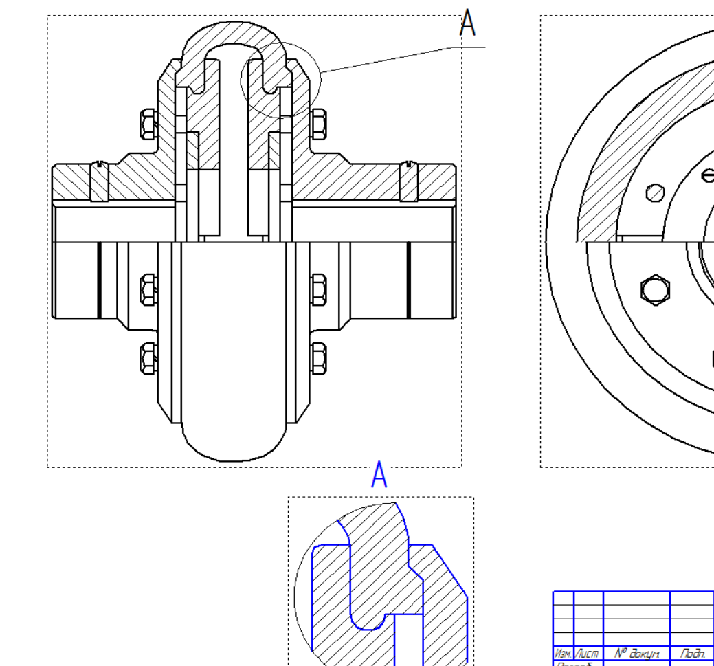
Рис. 4.10. Вид с выносным элементом
