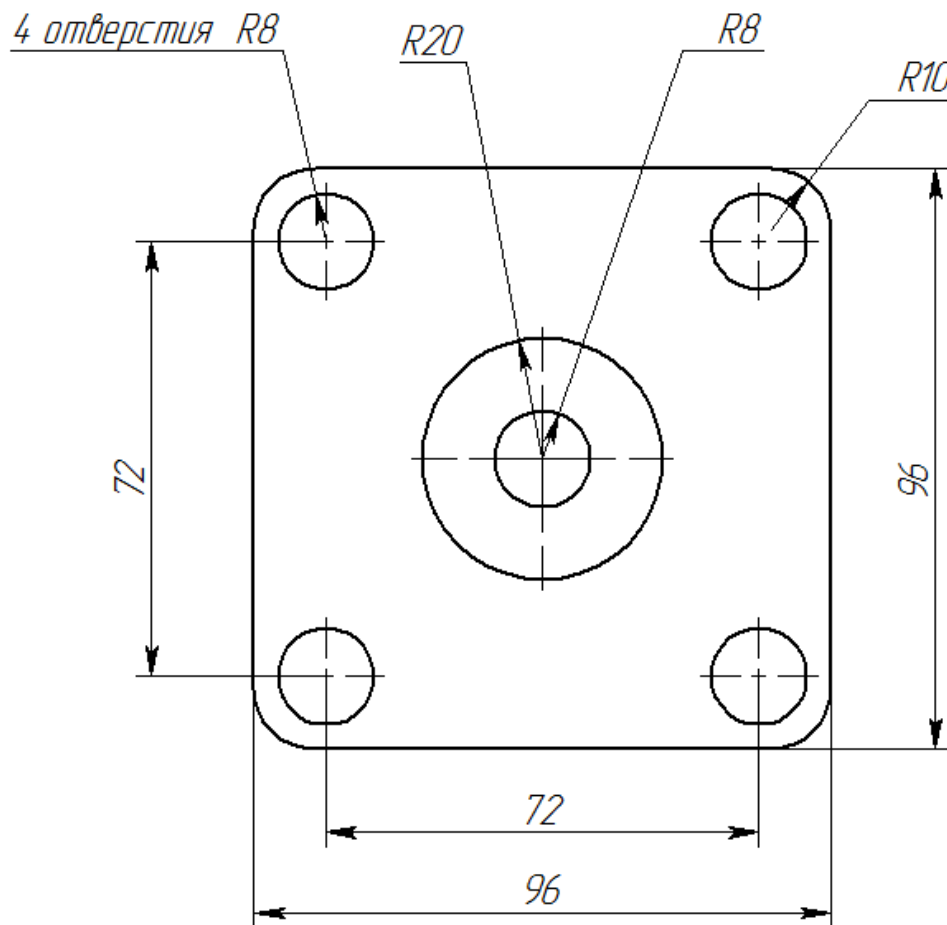
Рис. 7.1. Параметрическая 2D-модель
