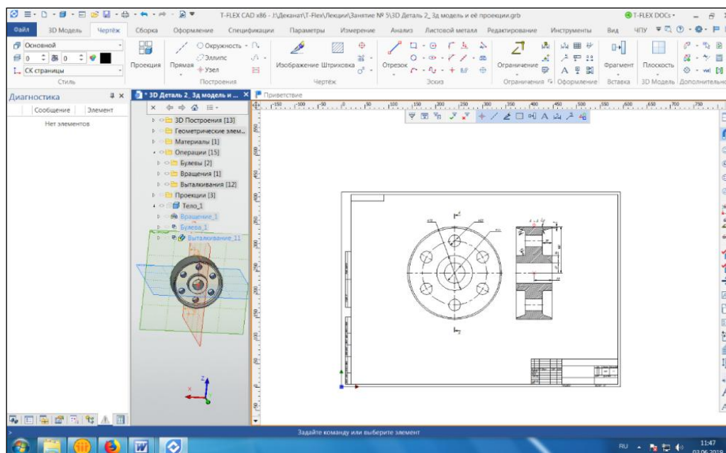
Рис. 9.10. Проекции Вид спереди и Вид справа
