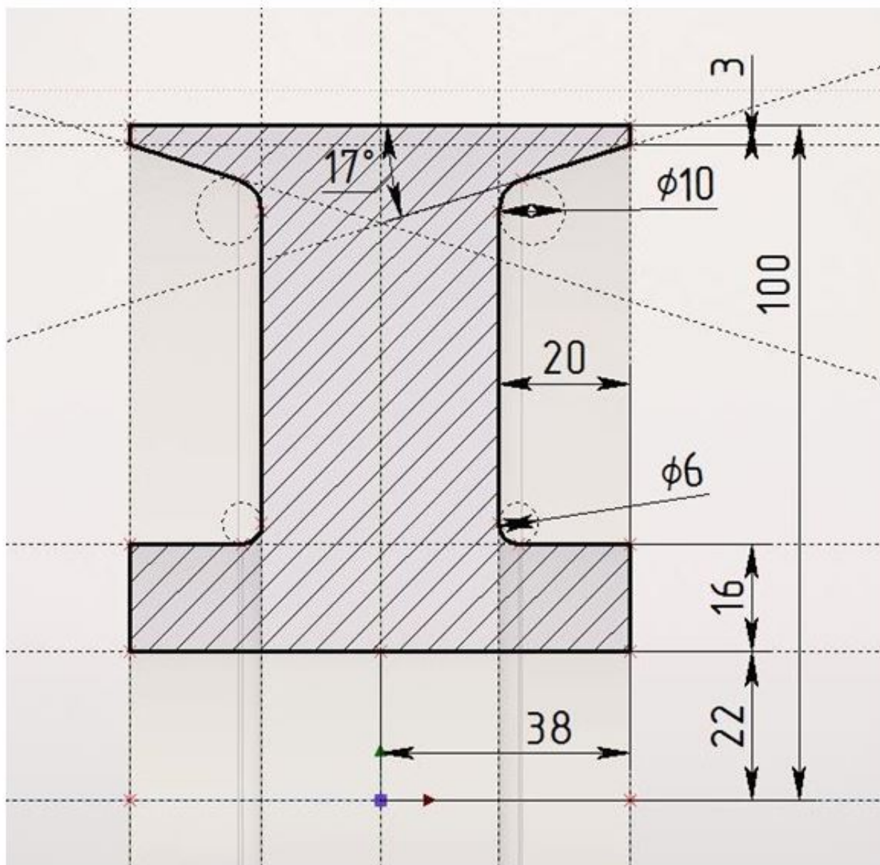
Рис. 9.4. Чертеж 3D-профиля на рабочей плоскости Вид спереди
