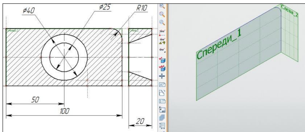
Рис. 8.10. 3D-профиль на рабочей плоскости Вид спереди
