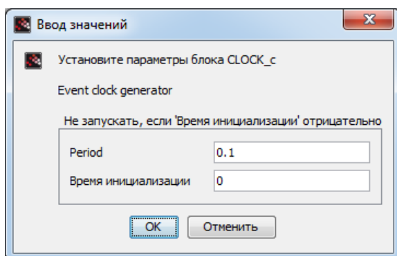
Рис. 1.3. Окна настройки параметров блоков CONST ( a ), BIGSOM_f ( б ), CLOCK_c ( в ), CSCOPE ( г ), примеры
