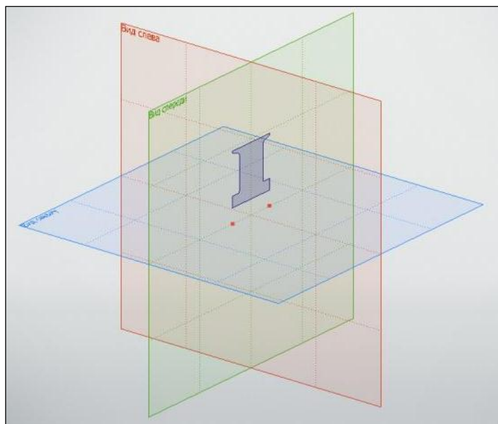
Рис. 9.5. 3D-профиль и 3D-узлы
