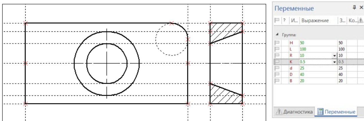
Рис. 8.6. Вид спереди, вид слева и окно Переменные
