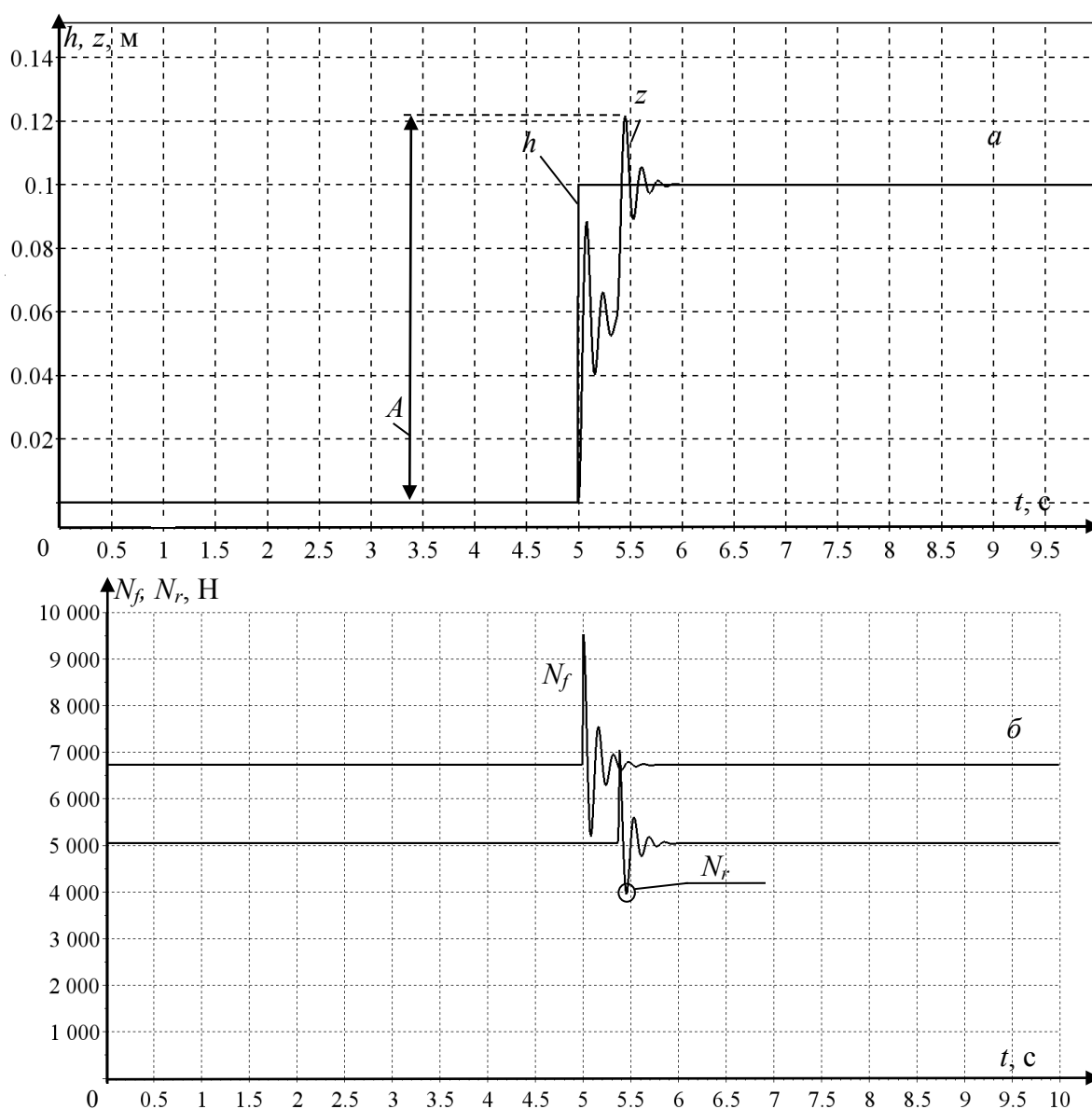
Рис. 2.3. Визуализация некоторых результатов моделирования (пример наезда машины на неровность высотой h = 0,1 м): a – линейное перемещение центра масс; \bar{b} – нормальные реакции на ходовых элементах
