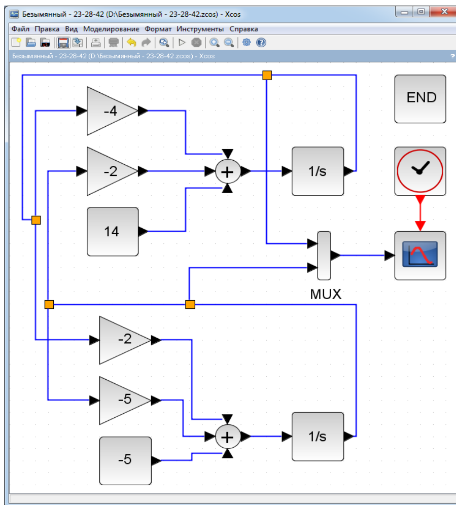
Рис. 1.5. Блочная диаграмма модели системы дифференциальных уравнений, эквивалентной системе линейных алгебраических уравнений второго порядка
