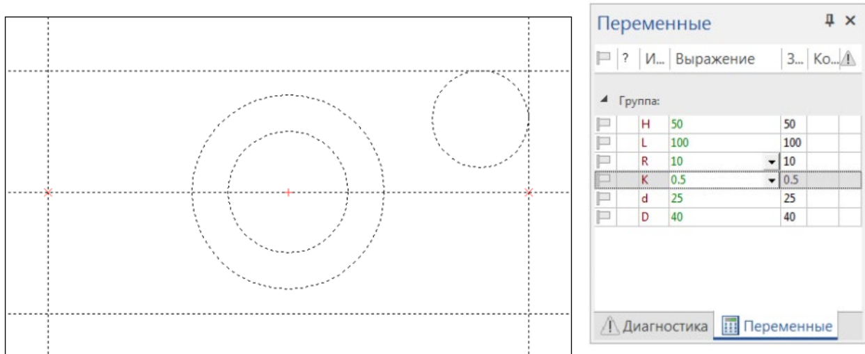
Рис. 8.5. Линии построения и окно Переменные
