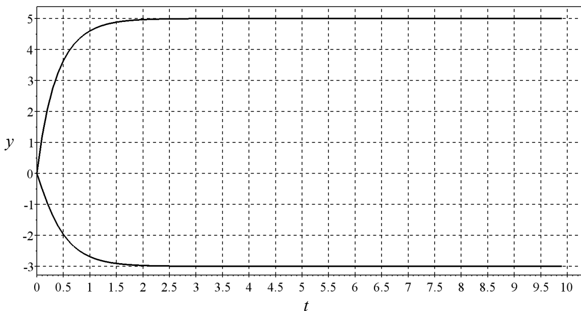
Рис. 1.6. Переходный процесс установления решения системы линейных алгебраических уравнений путем сведения к эквивалентной дифференциальной системе уравнений
