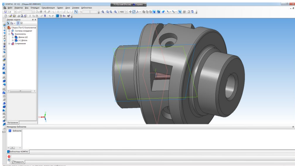
Рис. 6.2. Промежуточный этап совмещения деталей, при котором соблюдается соосность малых отверстий, но не соблюдается параллельность между плоскими гранями полумуфта
