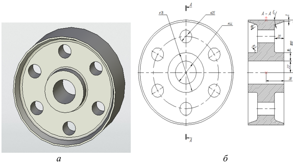
Рис. 9.1. 3D-модель (а) и ее проекции (б)
