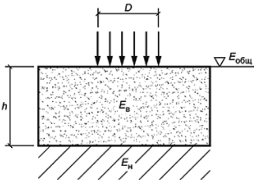
h - верхний слой конечной толщины; E_в - модуль упругости верхнего слоя; E_н - модуль упругости упругого полупространства, не ограниченного снизу (нижнего слоя); E_{общ} - модуль упругости на поверхности верхнего слоя
