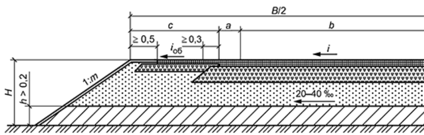
а - устройство дренающего слоя на всю ширину земляного полотна
