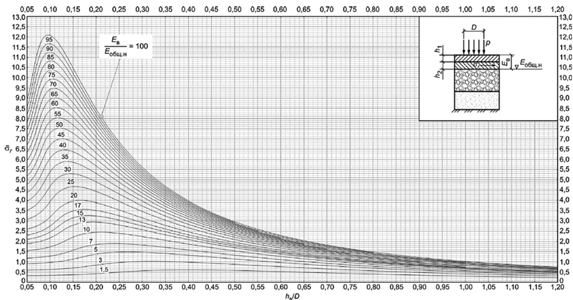
Рисунок Е.52 - Номограмма для определения растягивающего напряжения \bar{\sigma}_r при изгибе от единичной нагрузки в верхнем монолитном слое двухслойной системы при гладком контакте на границе слоев
