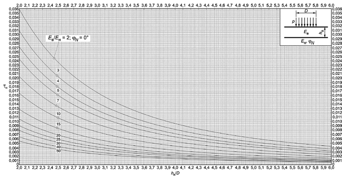
Рисунок Е.3 - Номограмма для определения единичного активного напряжения сдвига \tau_h от временной нагрузки в нижнем слое двухслойной системы при \varphi_N=0^\circ в диапазоне h_b / D=0,0-2,0
