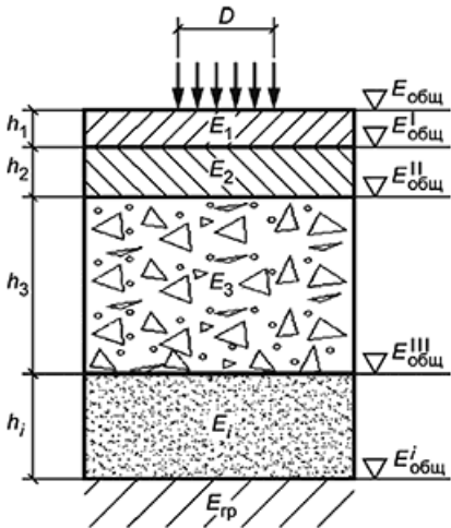
h_1, h_2, h_3, h_i - толщины слоев; E_{общ} - общий модуль упругости дорожной одежды; E_{общ}^I, E_{общ}^{II}, E_{общ}^{III}, E_{общ}^i - общие модули упругости на поверхности слоев; E_1, E_2, E_3, E_i - модули упругости материалов слоев; E_{гр} - модуль упругости грунта рабочего слоя
