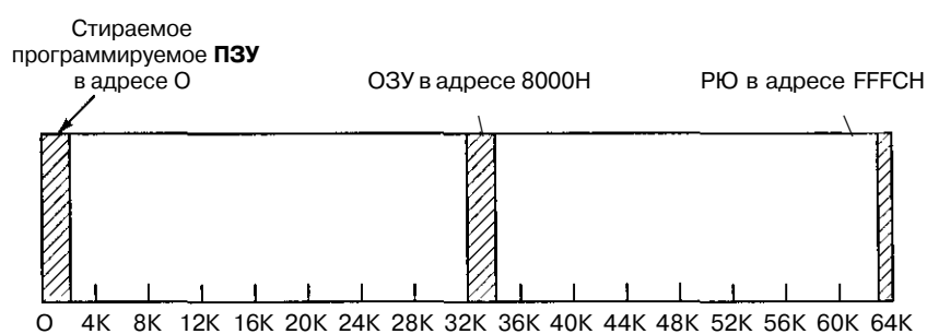
Рис. 3.52. Расположение стираемого ПЗУ, ОЗУ и РЮ на адресном пространстве в 64 К
