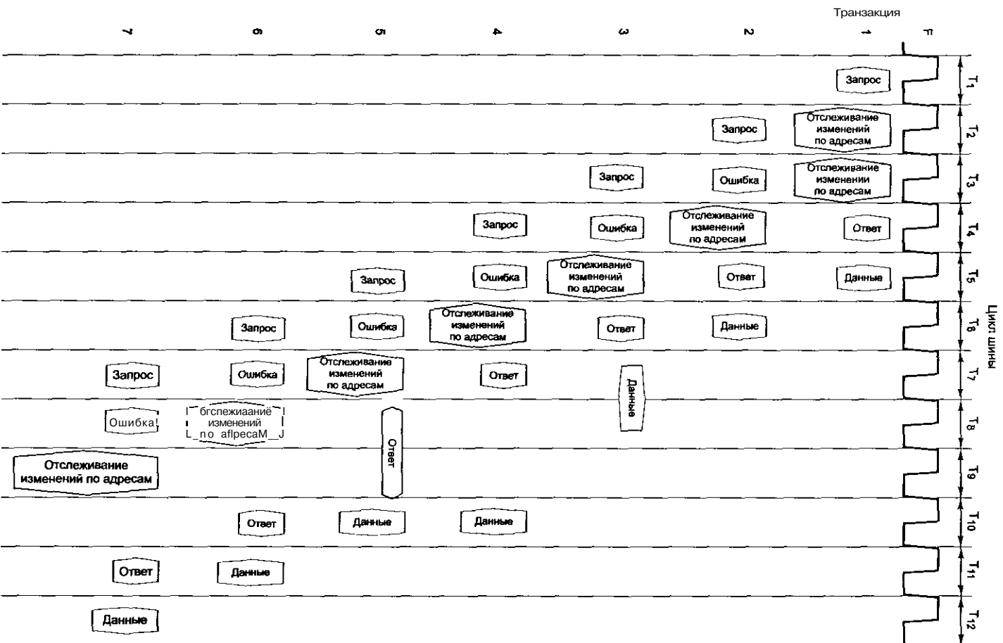
Рис. 3. Многоверный режим шины памяти в формате SDRAM
