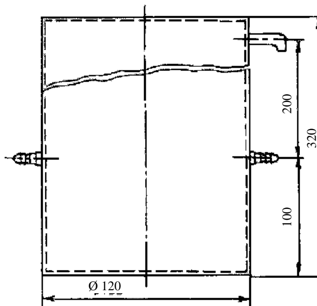
Рис. 2. Сосуд для отмучивания
