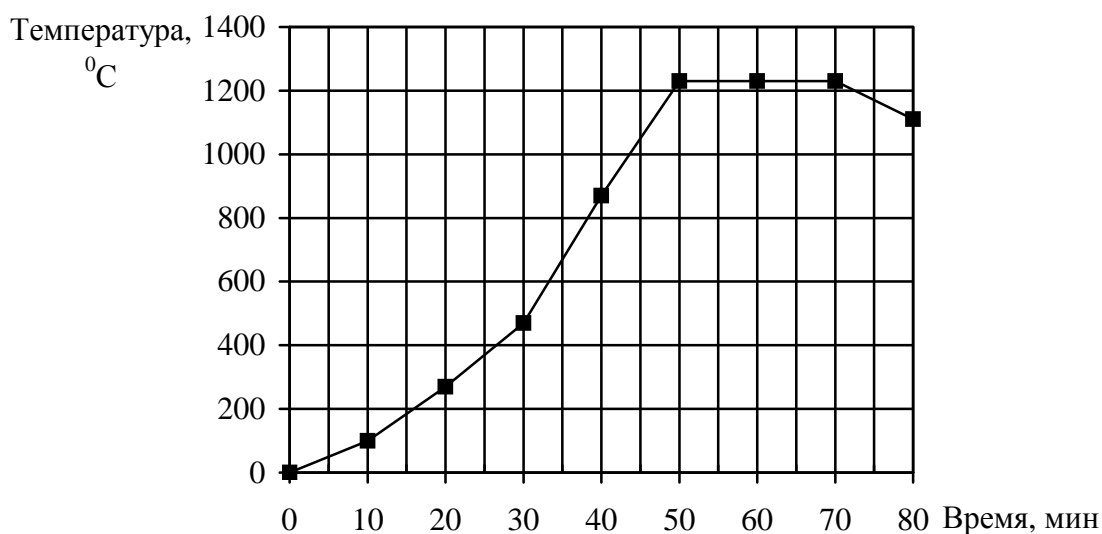
Рис. 8. Режим обжига сырьевых гранул
