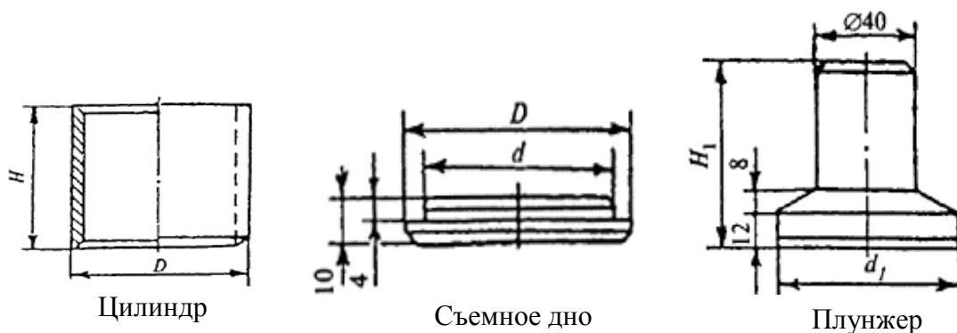
Рис. 5. Цилиндры стальные
