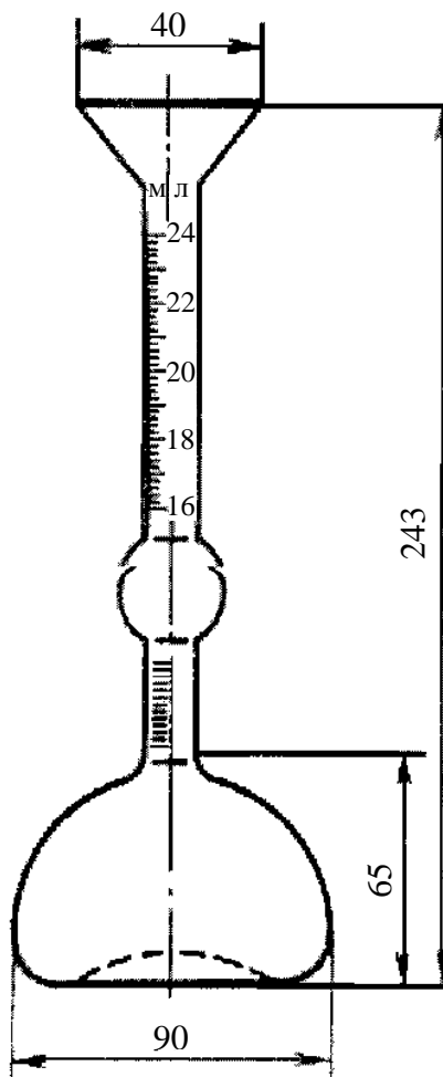
Рис. 3. Прибор Ле-Шателье
