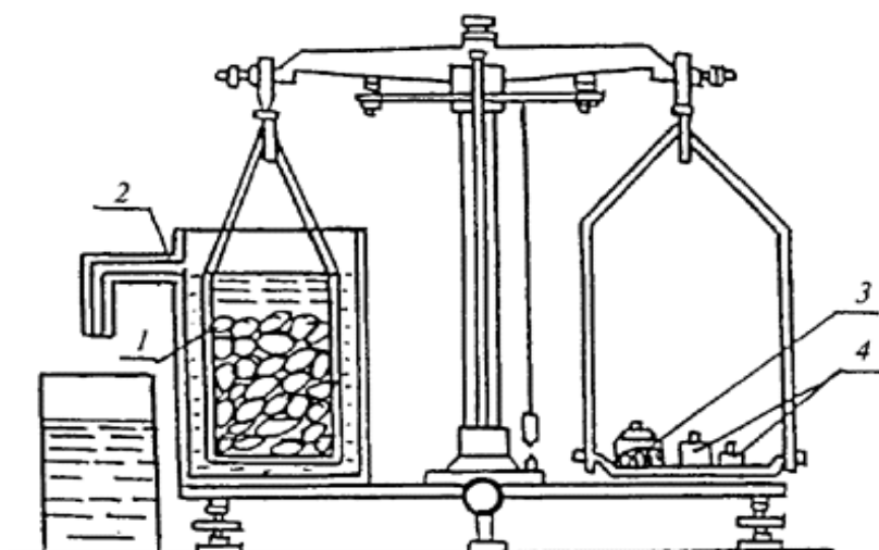
Рис. 7. Весы для гидростатического взвешивания: 1 – сетчатый (перфорированный) стакан; 2 – сосуд со сливом для воды; 3 – стаканчик с дробью для уравнивания массы сетчатого стакана в воде; 4 – разновесы
