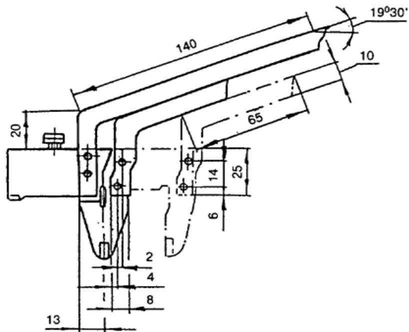
Рис. 4. Передвижной шаблон
