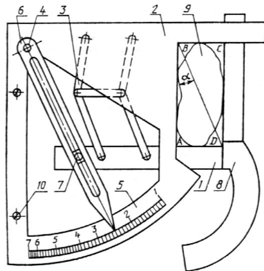
Рис. 9. Формомер:
