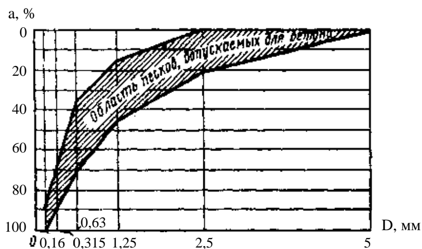
Рис. 1. Кривая просеивания песков:
