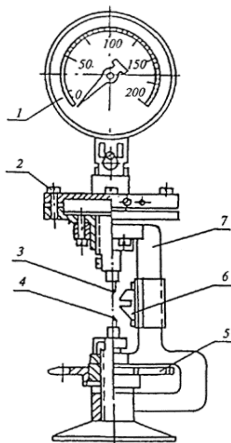
Рис. 6. Механический индикатор прочности камня (Т-3):
