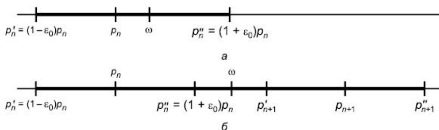
Рисунок 7.1 - Определение частот собственных колебаний
