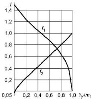
Рисунок 4.4 - График для определения коэффициентов f_1 и f_2
