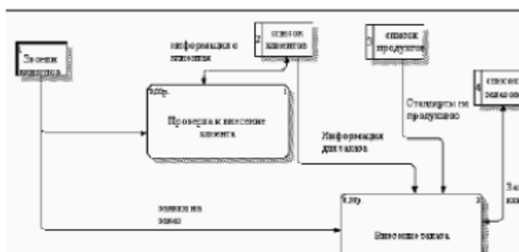
Рис. 8.9. Пример диаграммы DFD
