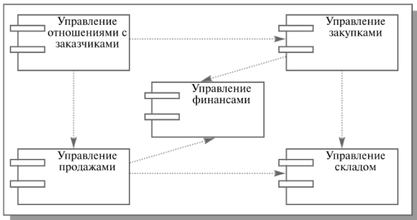
Рис. 11.9. Диаграмма компонентов фрагмента КИС
