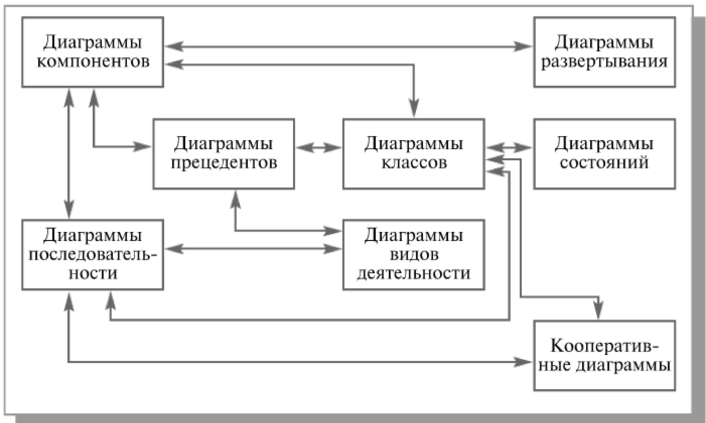
Рис. 12.1. Взаимосвязи между диаграммами UML
