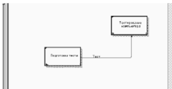
Рис. 7.19. Связь выход-механизм
