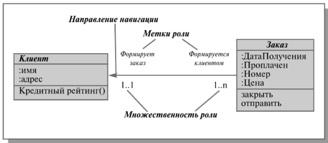
Рис. 11.3. Свойства ассоциации
