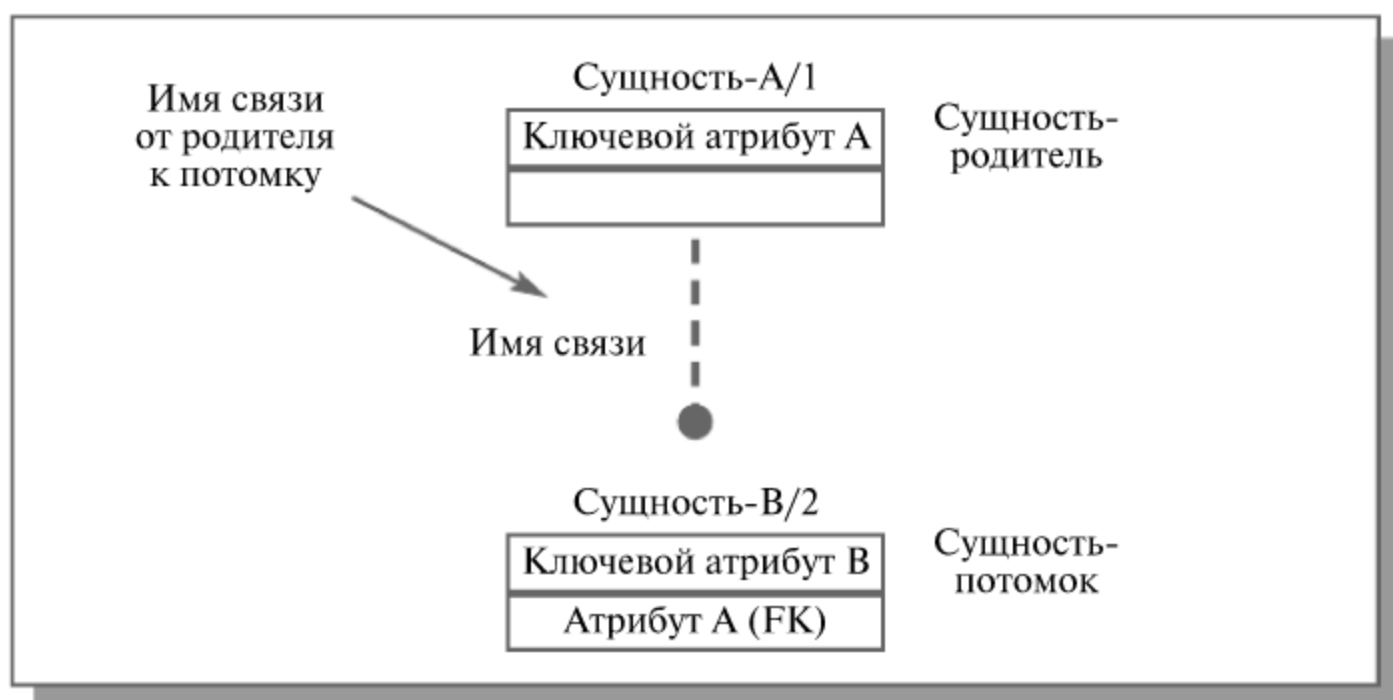
Рис. 10.4. Неидентифицирующая связь
