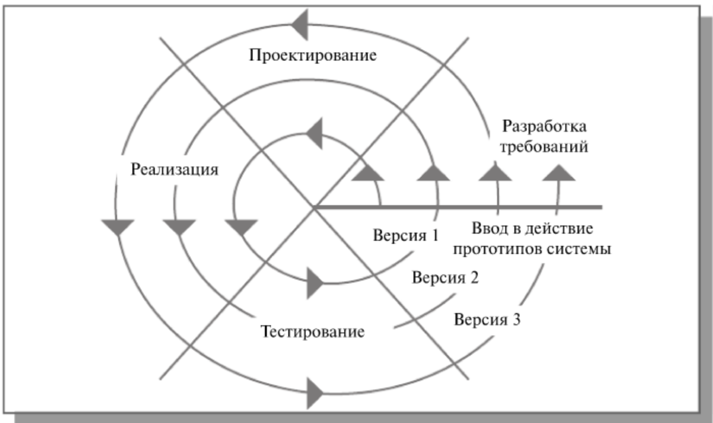
Рис. 2.3. Спиральная модель ЖЦ ИС
