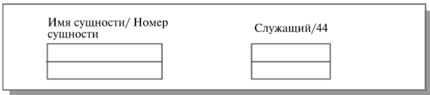
Рис. 10.1. Независимые от идентификации сущности
