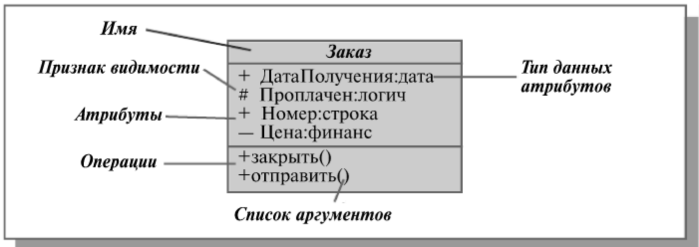
Рис. 11.1. Изображение класса в UML
