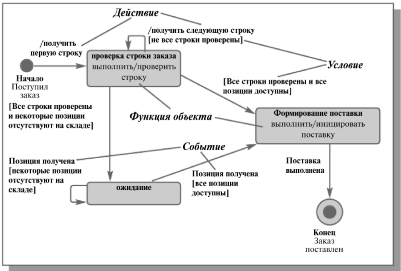
Рис. 11.7. Диаграмма состояний объекта «заказ»
