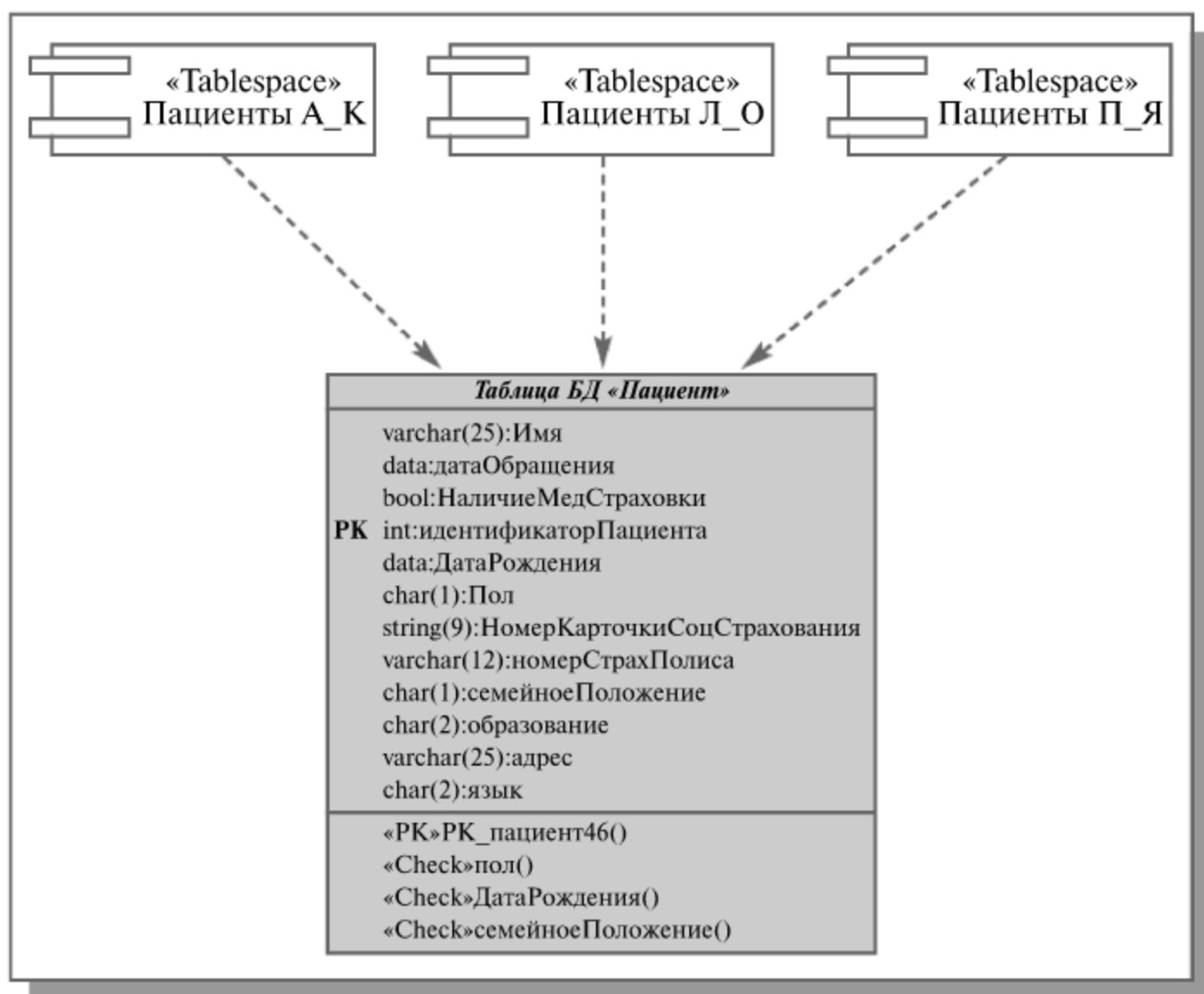
Рис. 12.15. Экстенды таблицы «Пациент»
