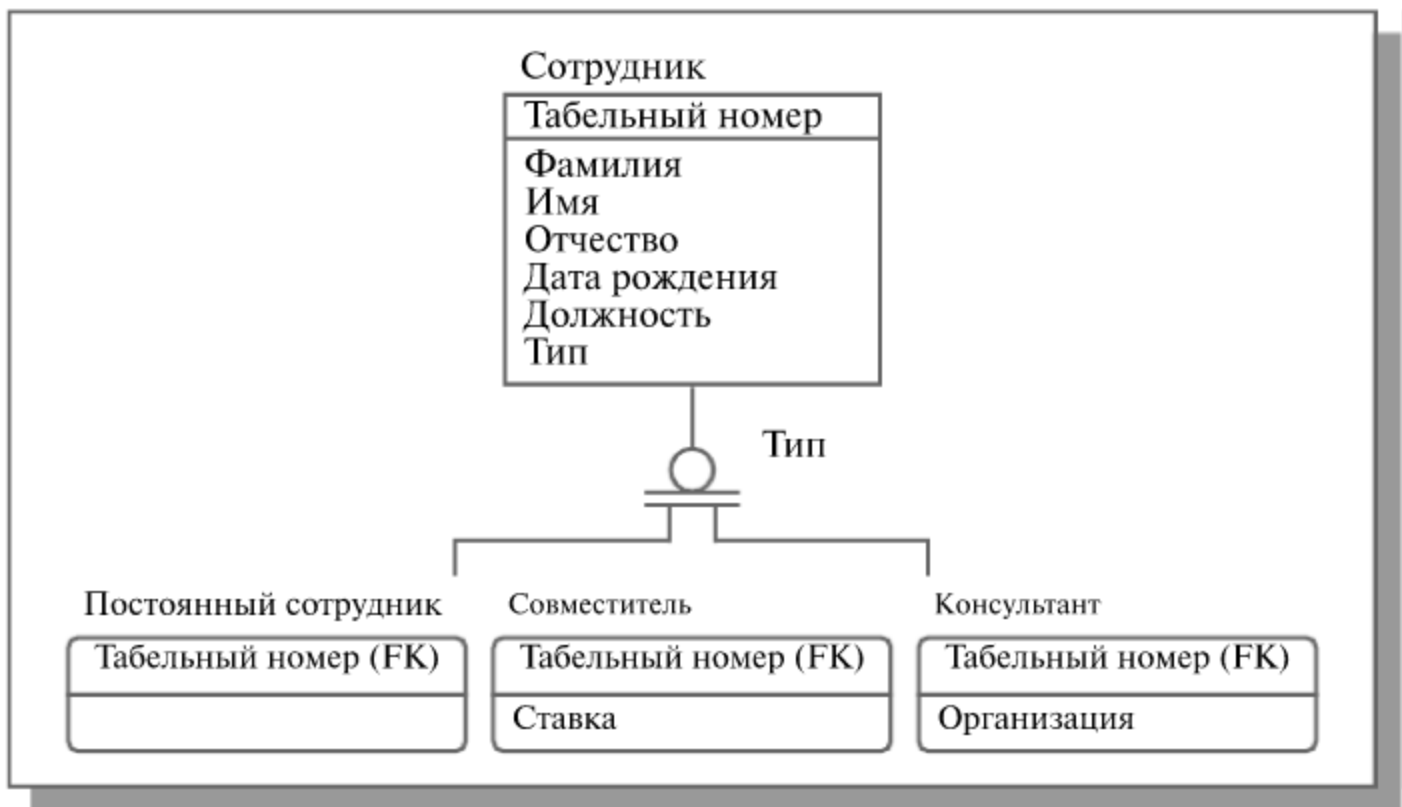
Рис. 10.9. Иерархия наследования. Полная категория
