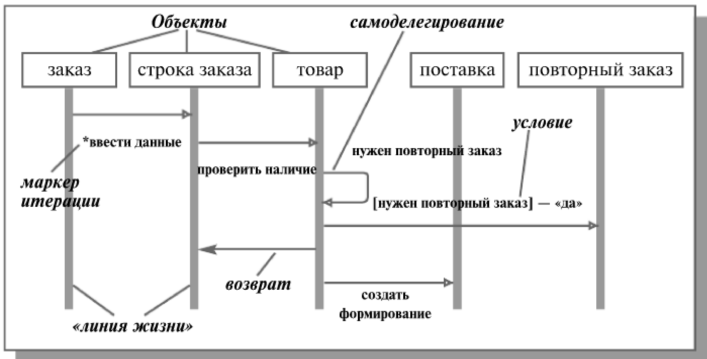
Рис. 11.5. Диаграмма последовательности обработки заказа:
