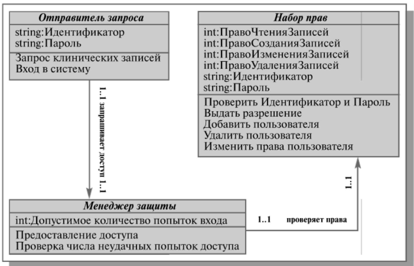
Рис. 12.11. Диаграмма классов «Защита доступа»
