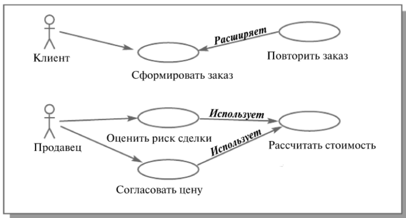
Рис. 11.4. Связи на диаграммах прецедентов
