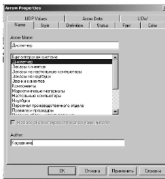
Рис. 7.11. Диалог IDEF0 Arrow Properties
