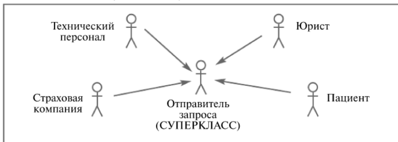
Рис. 12.6. Обобщение классов
