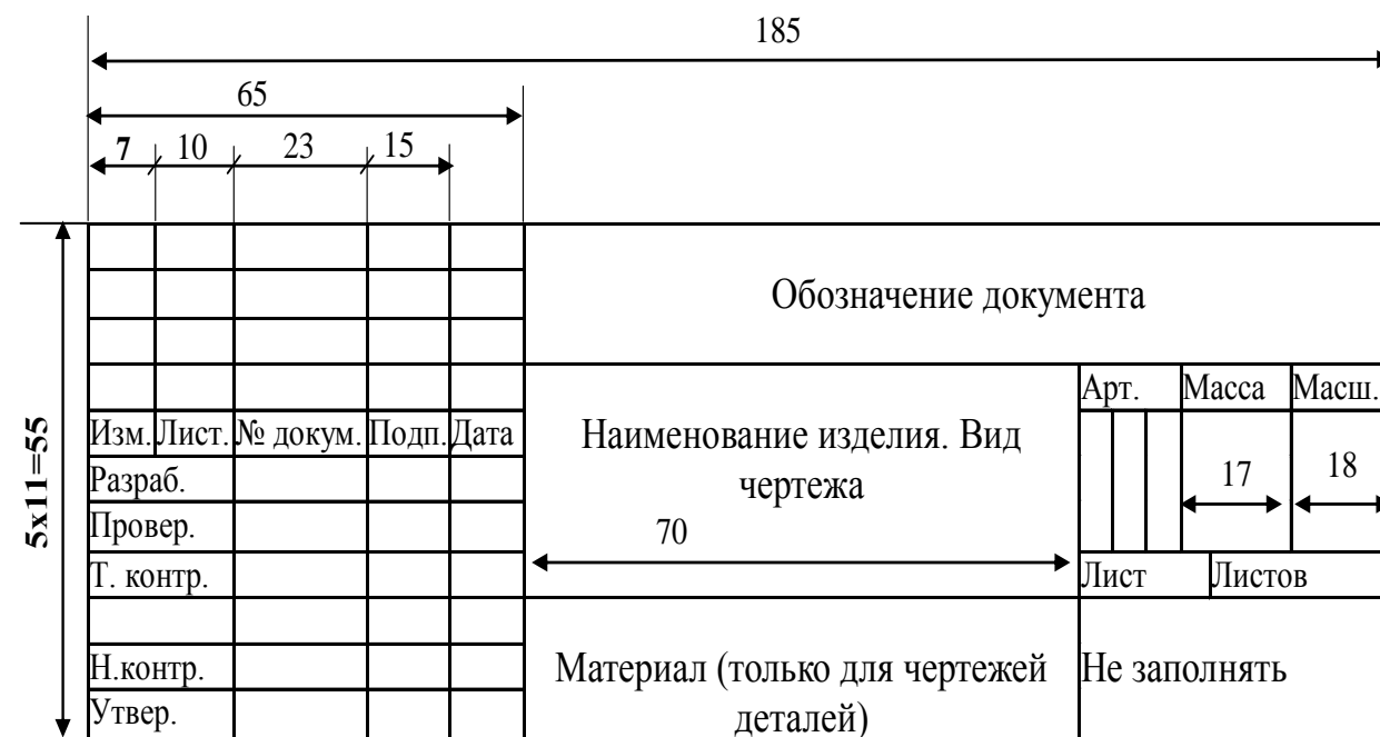
Рисунок 5.2 – Угловой штамп для чертежей деталей и схем
