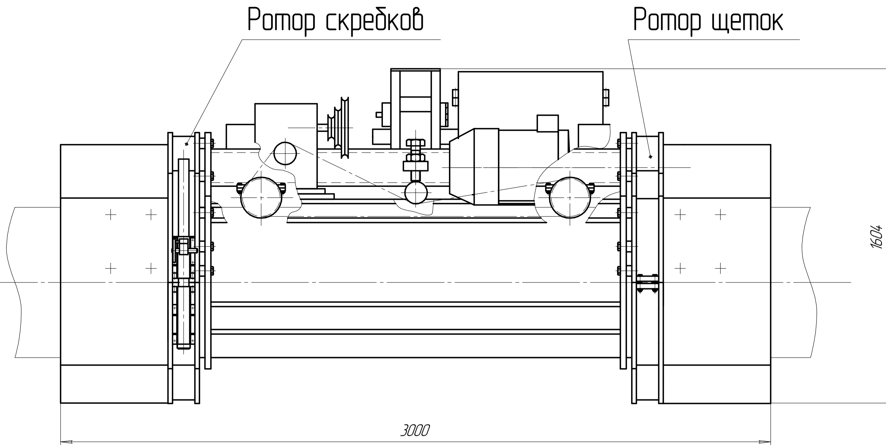
Привод ротора
