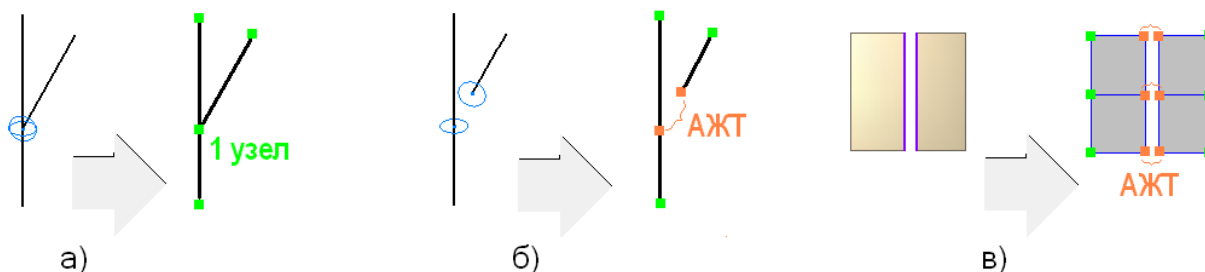
Рис. 8.13 Согласование сеток конечных элементов
