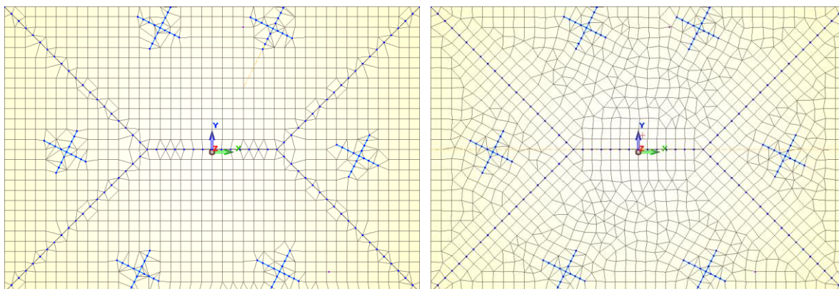
Рис. 8.15 Настройки триангуляции и результат генерации различных сеток: треугольной, четырехугольной и адаптивной четырехугольной.
