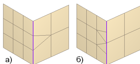
Рис. 8.17 Триангуляция в порядке а) от меньшего шага к большему б) от большего шага к меньшему
