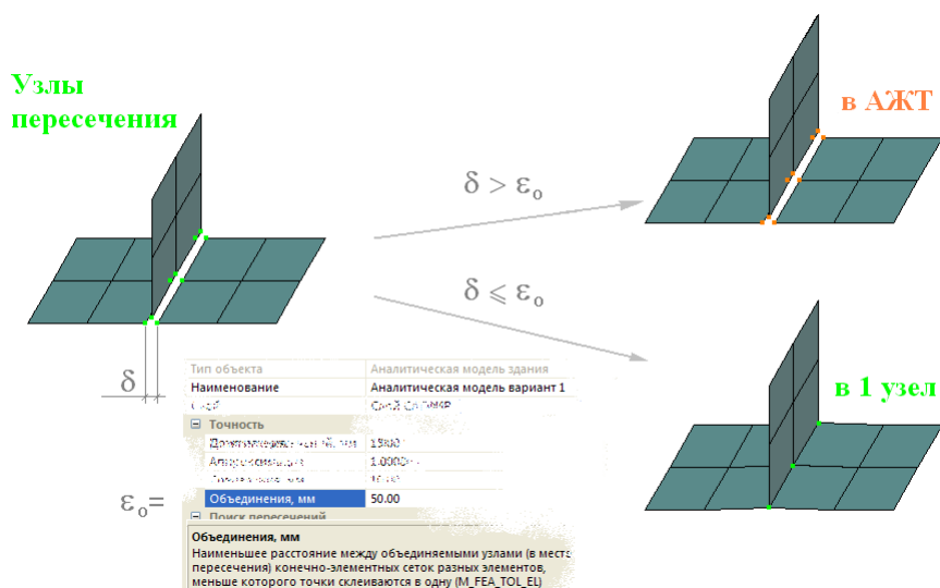
Рис. 8.22 Расчетная схема ПК ЛИРА на пересечении пластин
