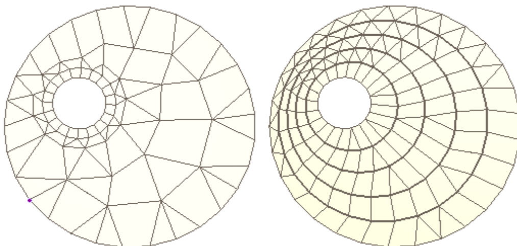
Рис. 8.9 Автоматическая триангуляция – слева и триангуляция с нанесением дополнительных отрезков – справа
