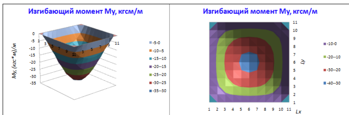
Рис.3.10. Эпюра изгибающего момента M_y
