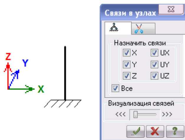
Рис. 4.14. «Жесткая» заделка
