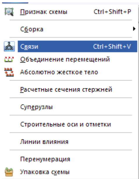
Рис. 4.12. Меню «Схема»
