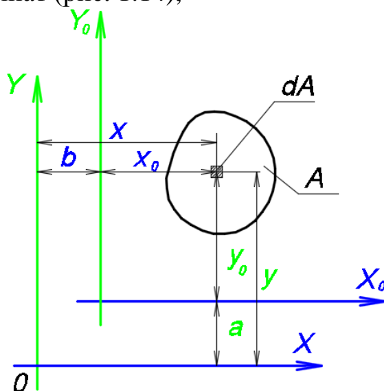
Рис. 1.14. Момент инерции относительно параллельных осей
