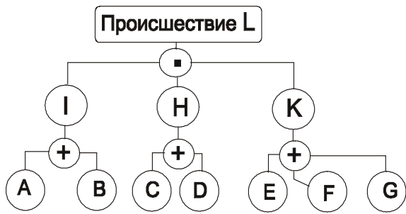
Дерево происшествия
