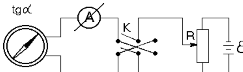
Рис. 4.2. Электрическая схема к лабораторной установке
