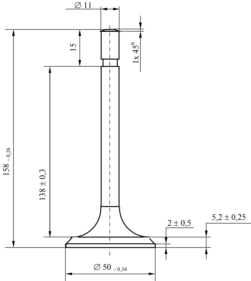
Рис. 1. Клапан
