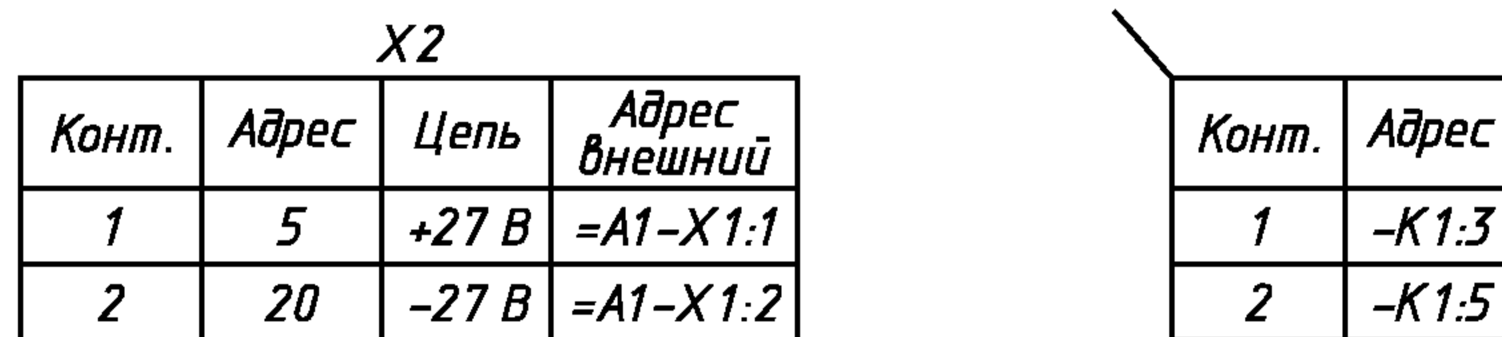
а – таблица, помещаемая на свободном поле схемы или на последующих листах схемы
