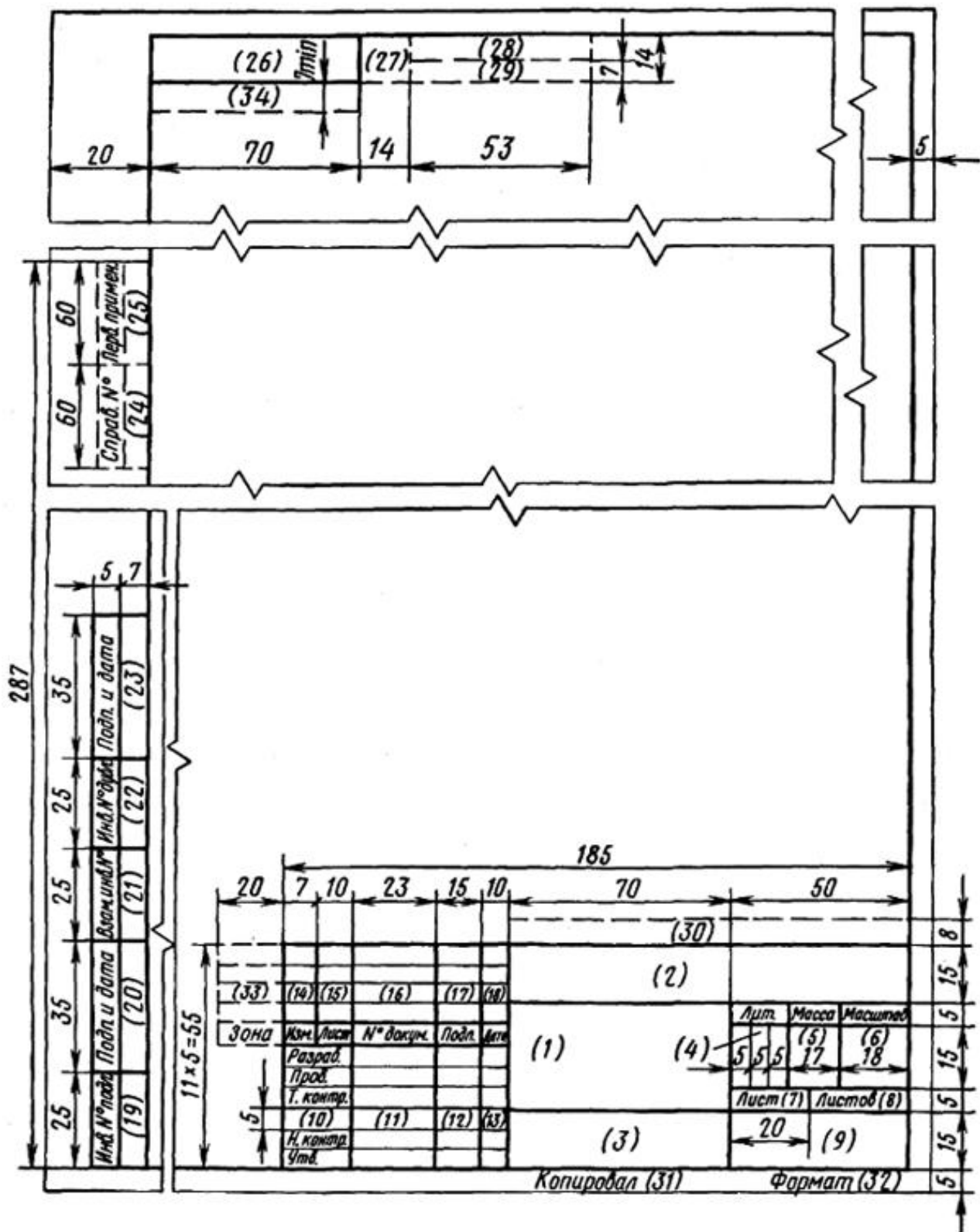
Форма 2. Основная надпись и дополнительные графы для текстовых конструкторских документов (первый или заглавный лист)
