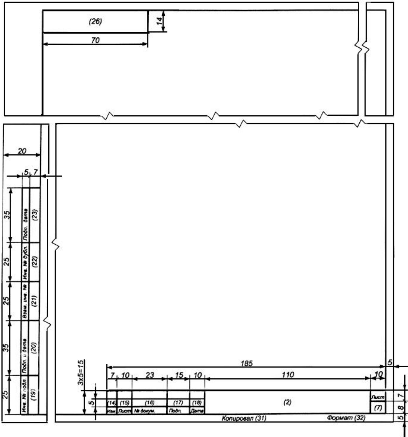
Форма 2б. Основная надпись и дополнительные графы для текстовых конструкторских документов при двустороннем светокопировании (последующие листы)
